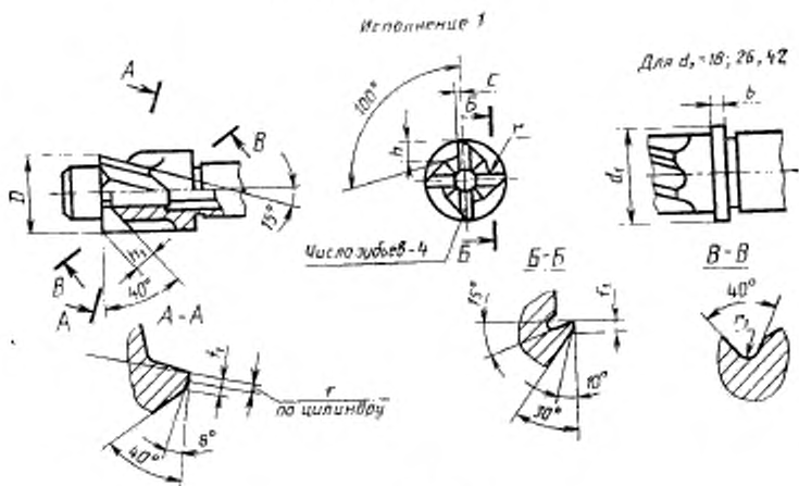
Тип 4 (черт. 11, табл. 13)
