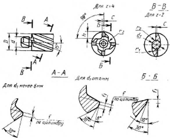
Тип 1 (черт. 8, табл. 10)
