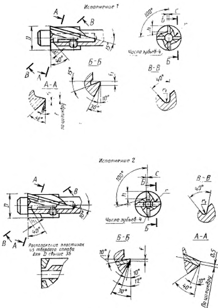
Тип 2 (черт. 9, табл. 11)
