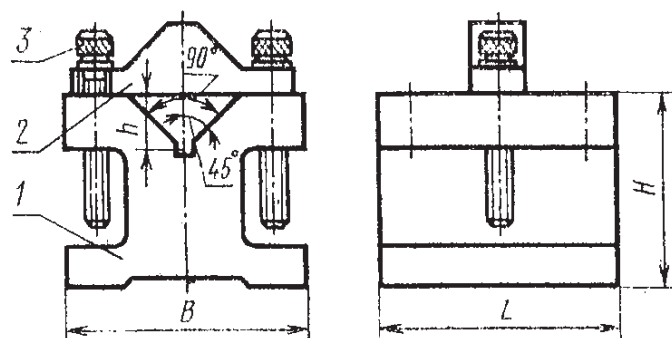
1—корпус призмы; 2—накладка; 3—винт крепления накладки.
