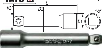
Подовжувач похилений
