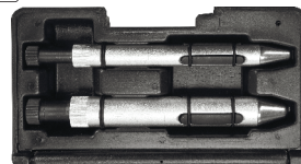
Набір для центрування дисків зчеплення в межах Ø= 15-20 мм і Ø= 20-27 мм 2 елем.
