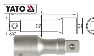
Подовжувач
