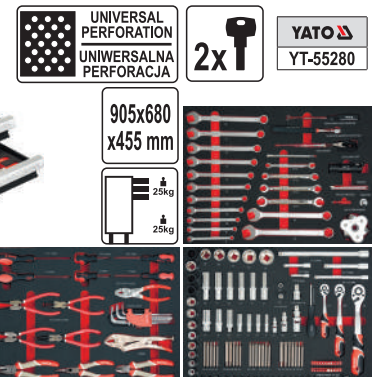
Шафа з інструментами 162 елем., 3 шухляди
