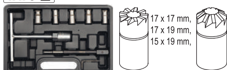
Фрези для гнізд сопл форсунок 7 шт.
