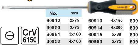
Викрутка "Cushion Grip" пряма
