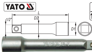
Подовжувач
